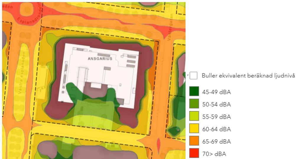
Bullerkartering 2019, ekvivalent ljudnivå, Växjö kommun
