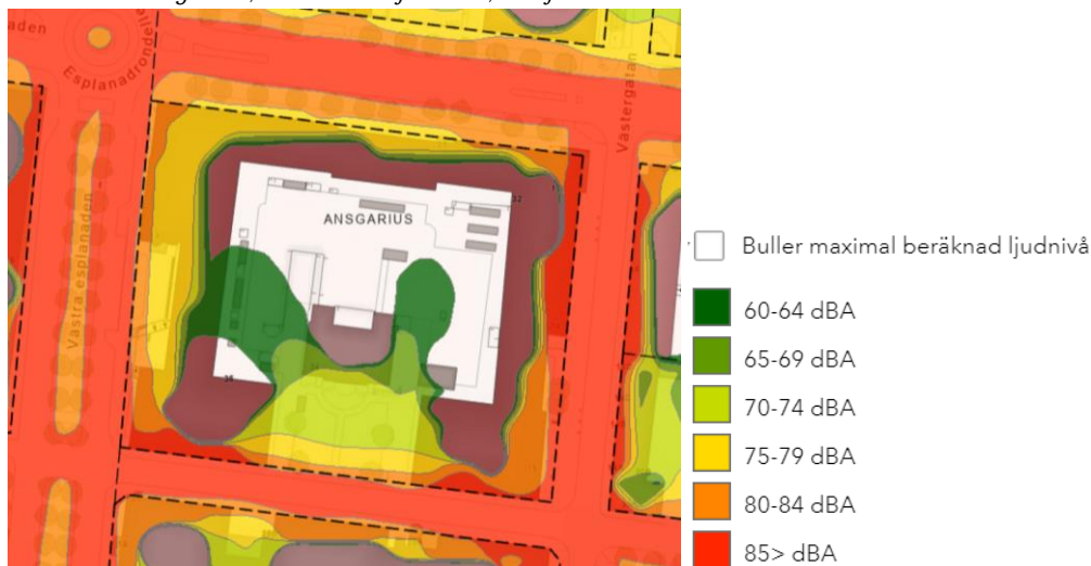
Bullerkartering 2019, maximal ljudnivå, Växjö kommun
